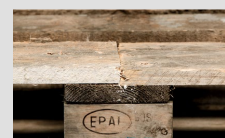
Επισκευή που δεν συμμορφώνεται με τις προδιαγραφές
