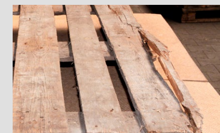
Σπασμένες εγκάρσιες σανίδες μερικώς ή εντελώς σπασμένες σανίδες
